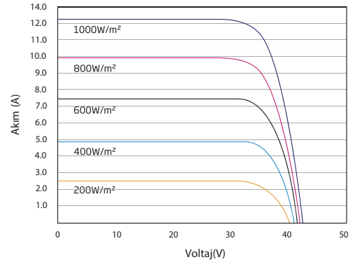
Akım - Voltaj Grafiği (TT400-120TPM12)
